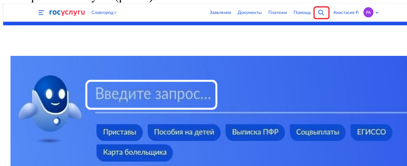
Рисунок 1. Поиск услуги
